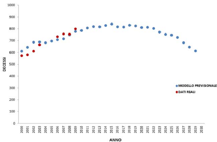
Fig. 2. Numero di decessi per mesotelioma maligno della pleura negli uomini e decessi stimati mediante il modello previsionale basato sui consumi di amianto in Italia (Marinaccio et al, 2005).
